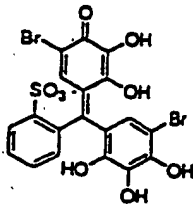
BROMOPYROGALLOL RED
